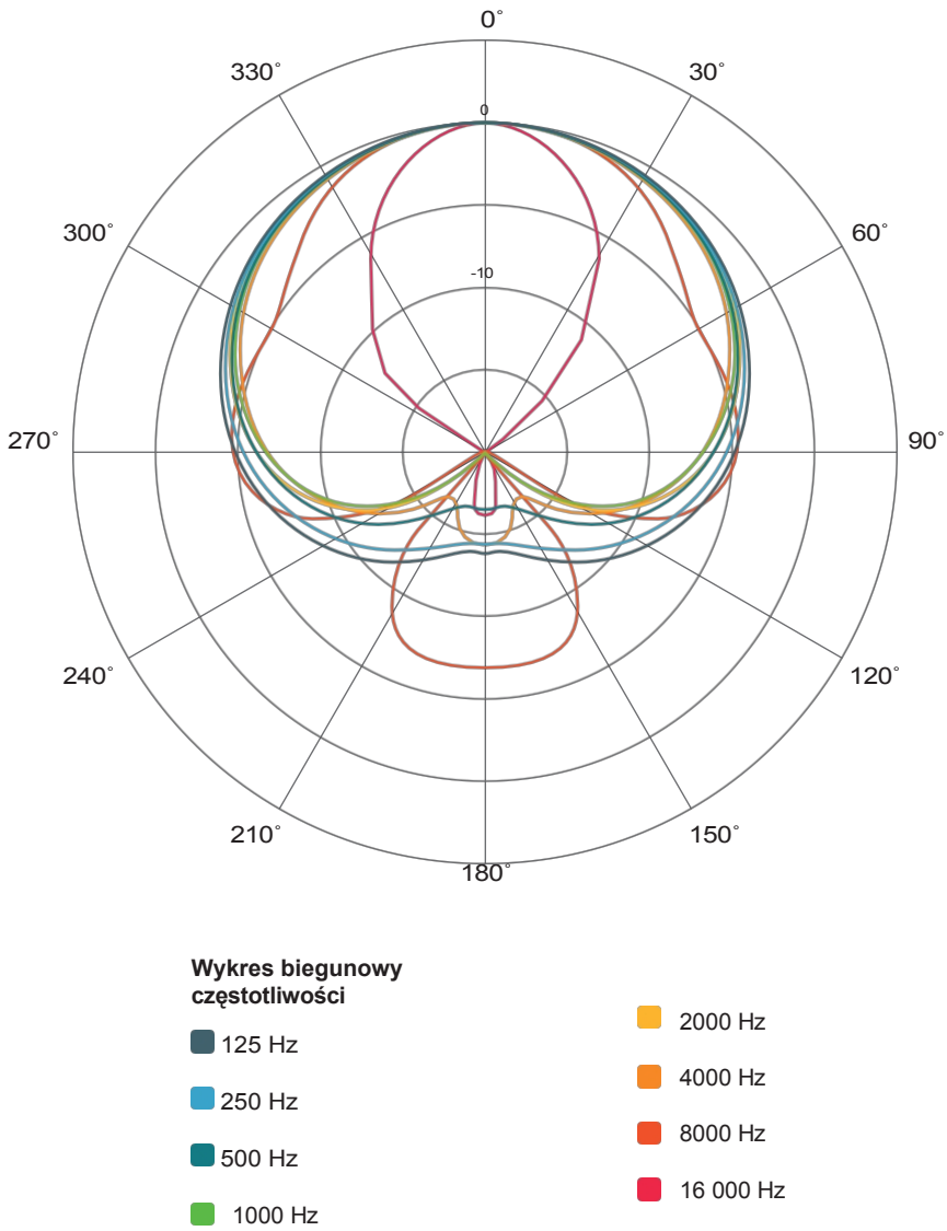
Rysunek 9.2 – Wykres polarny urządzenia LCT 440 PURE
