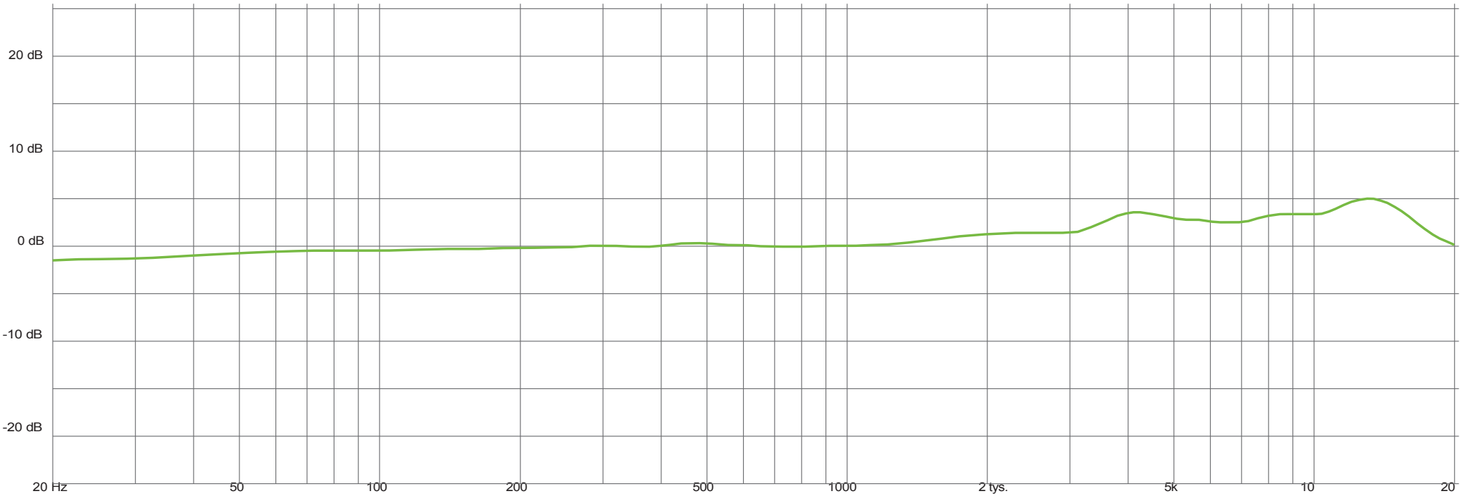
Rysunek 9.1 – Charakterystyka częstotliwościowa LCT 440 PURE
