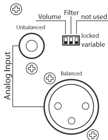
Złącza tylne i przełączniki DIP
